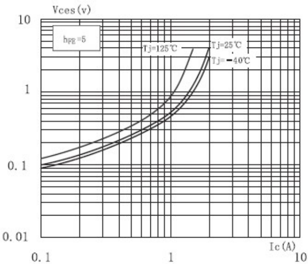
V_{ces} - I_c
