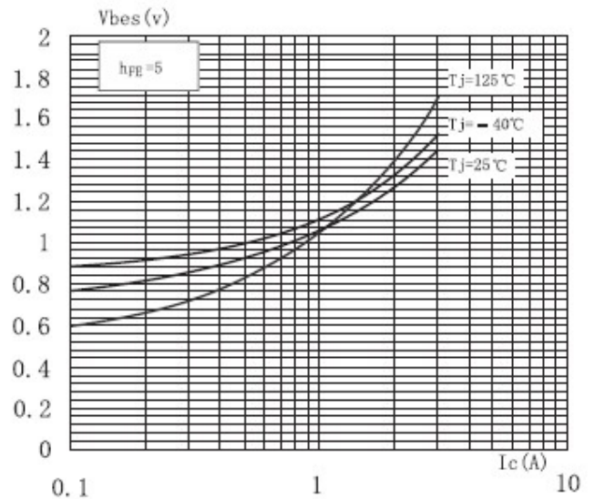
V_{bes} - I_c
