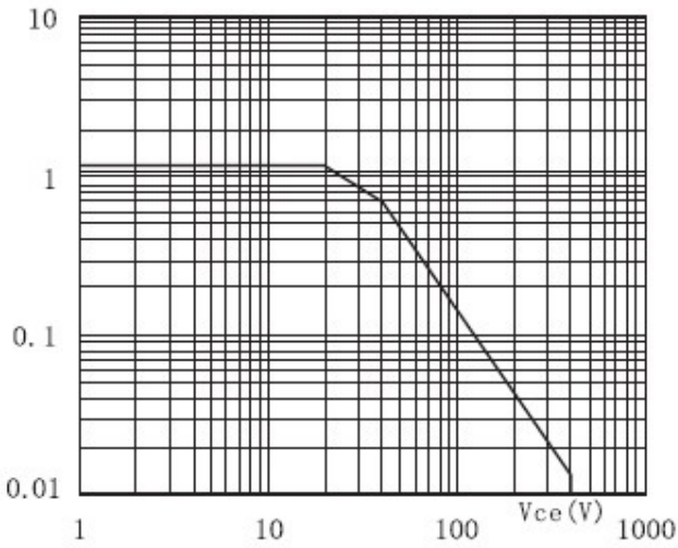
SOA (DC)
